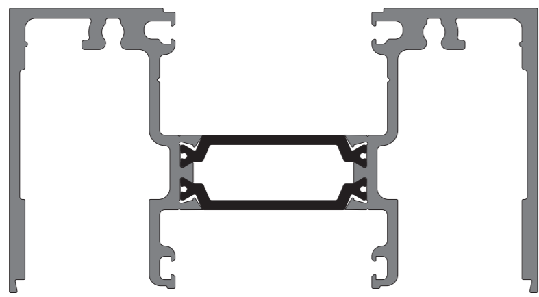
KAS 721 Mullion
