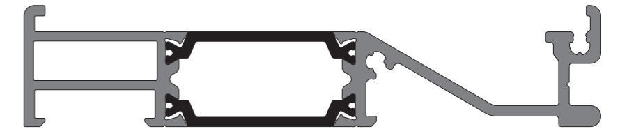
KAS 725 Subcill
